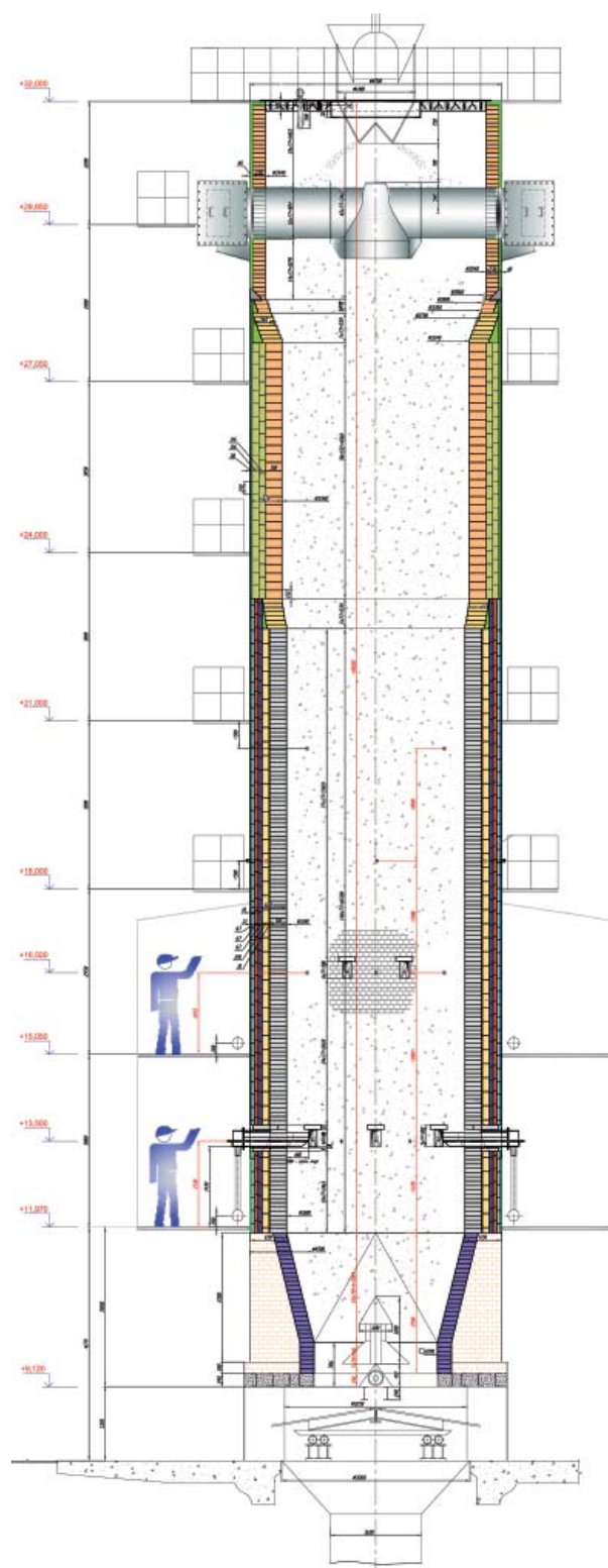
Рис. 1. Противоточная шахтная печь
